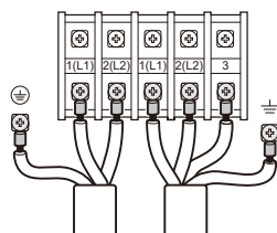
Câble d'alimentation électrique
