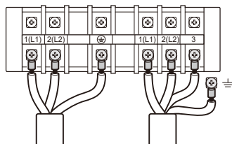
Câble d'alimentation électrique
