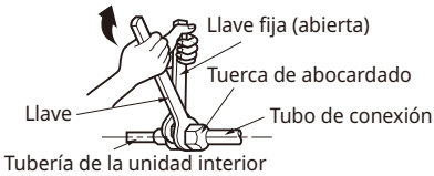
Para multizona ODU
