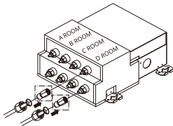
(Sólo unidades interiores de 36 kBtu/h – conectar “D ROOM”)
