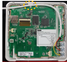
Le bossage central supérieur pour la fixation du câble plié
