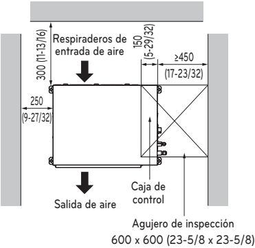
Vista superior [Unidad: mm(inch)]
