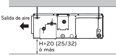
Vista lateral [Unidad: mm(inch)]
