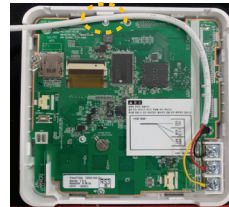
Retén central superior para fijar el cable doblado
