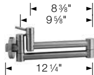
BLANCO CANTATA™ Pot filler
