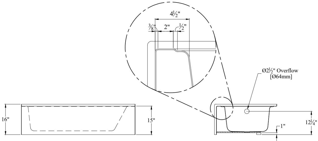
ELEVATION
