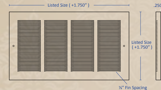
Model 173 • 1/3" Fin Spacing
