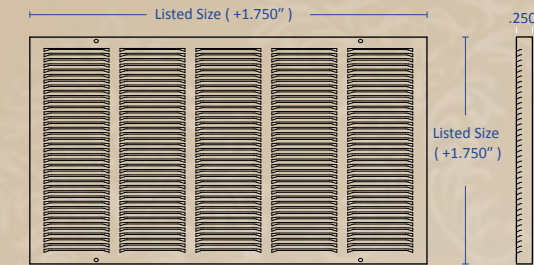
Model 170 • 1/2" Fin Spacing
